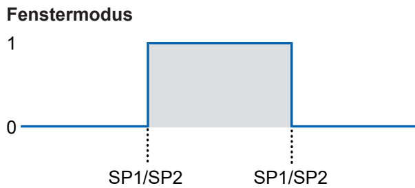
Abb. 7: Sensor im Schaltmodus Fenstermodus
