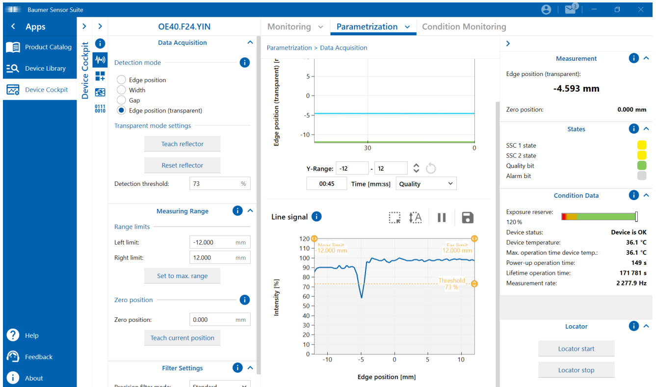
Abb. 2: Einstellungen für Edge position (transparent) am Beispiel BSS
