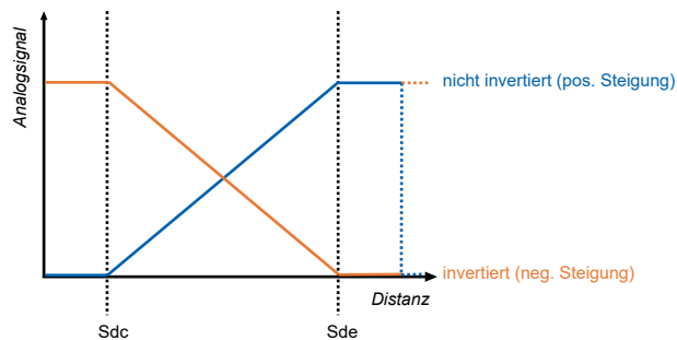
Abb. 13: Analogausgang – Invertiert
