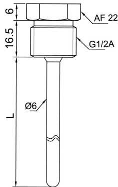
G 1/2 A ISO 228-1 (BCID: G06)
